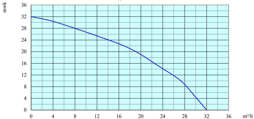
Q-H kromme
