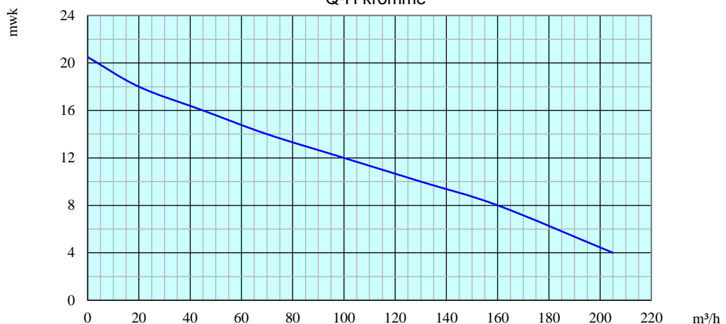
Q-H kromme
