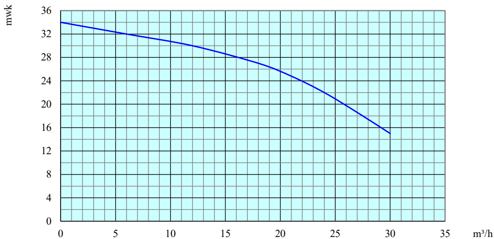
Q-H kromme
