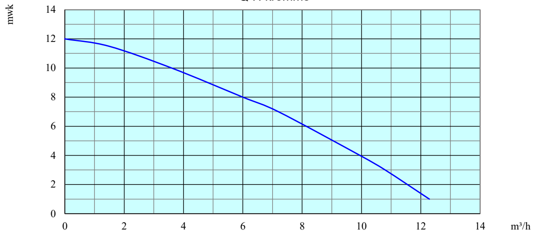
Q-H kromme
