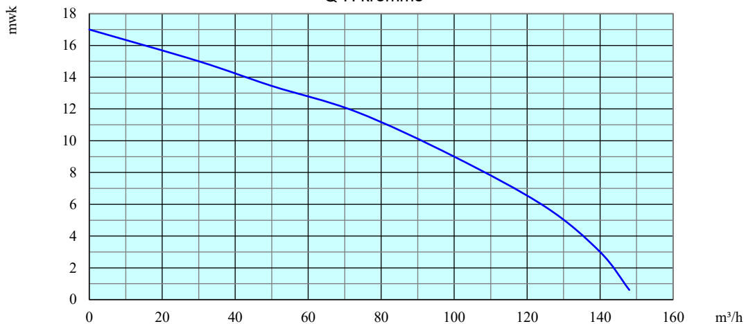
Q-H kromme
