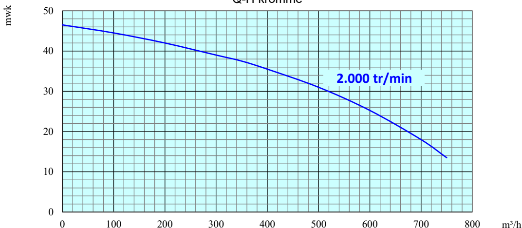
Q-H kromme
