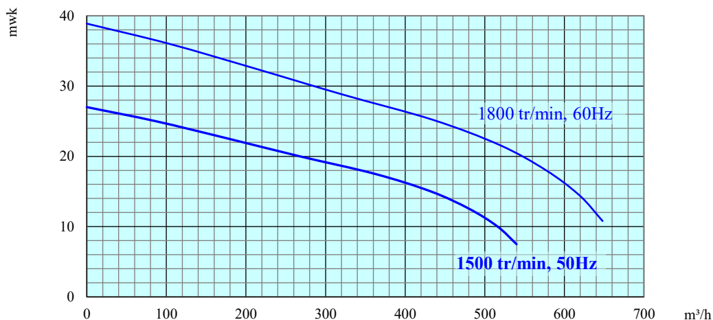
Q-H kromme
