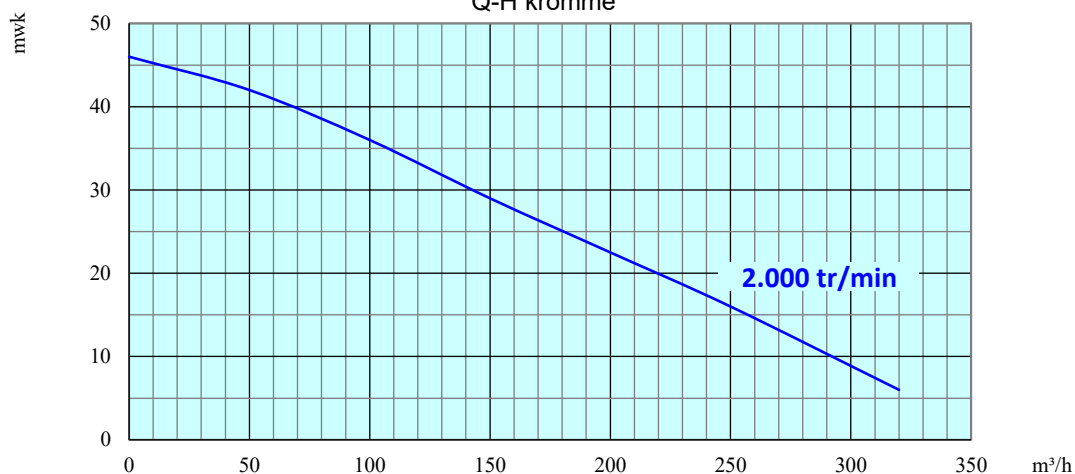
Q-H kromme
